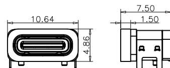
加防水圈示意图
